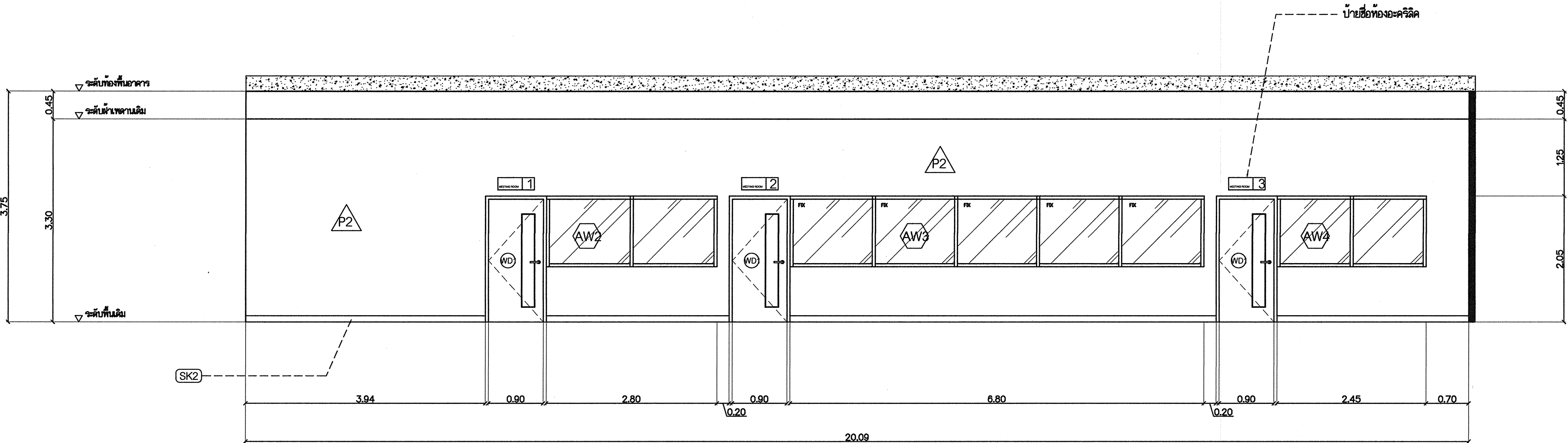
รูปด้าน A SCALE : 1:50
