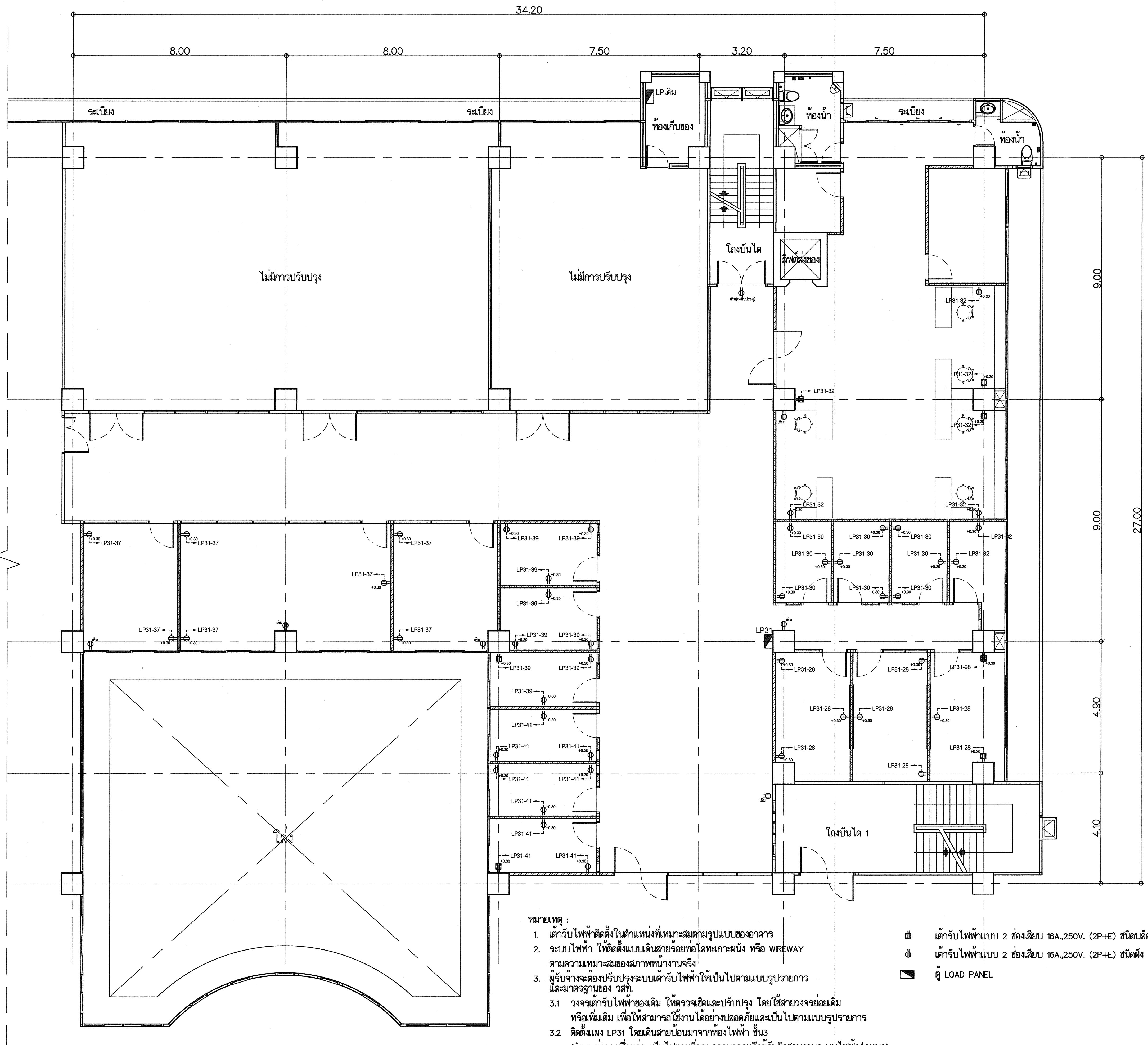
แปลนระบบเตาไฟฟ้า ชั้น3R (หลังปรับปรุง) SCALE : 1:75
