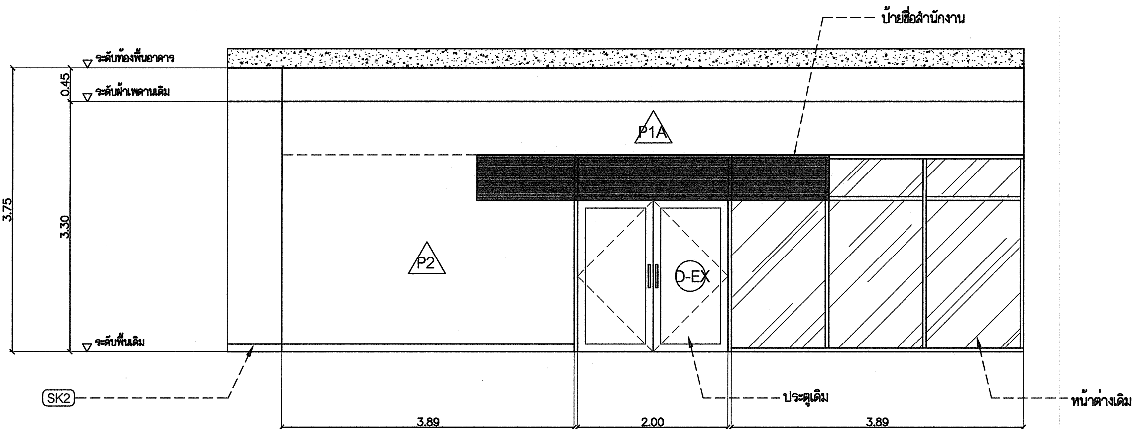
รูปด้าน E SCALE : 1:50
