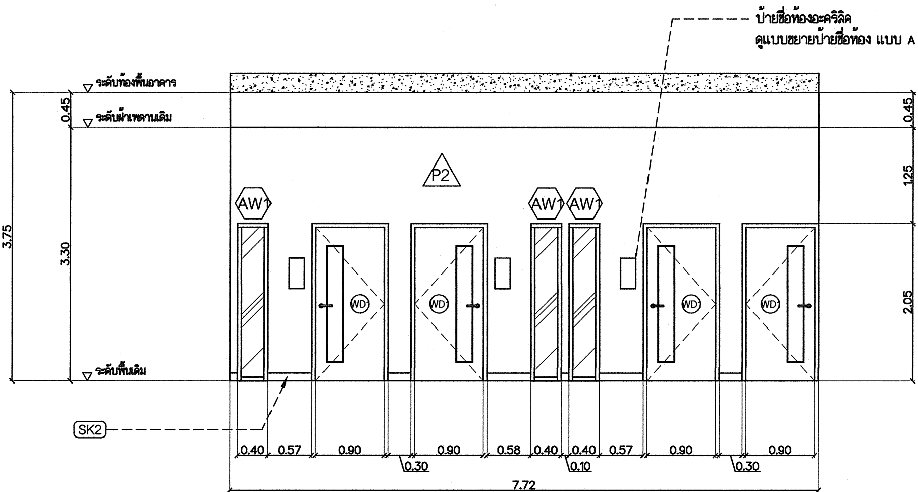
รูปด้าน C SCALE : 1:50
