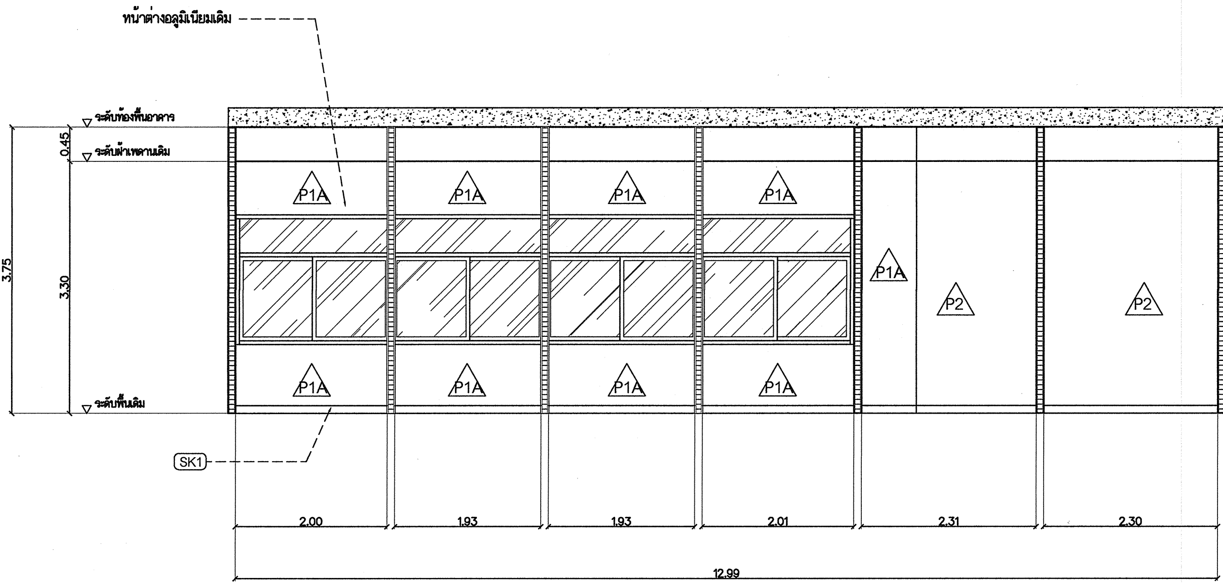
รูปตัด B
