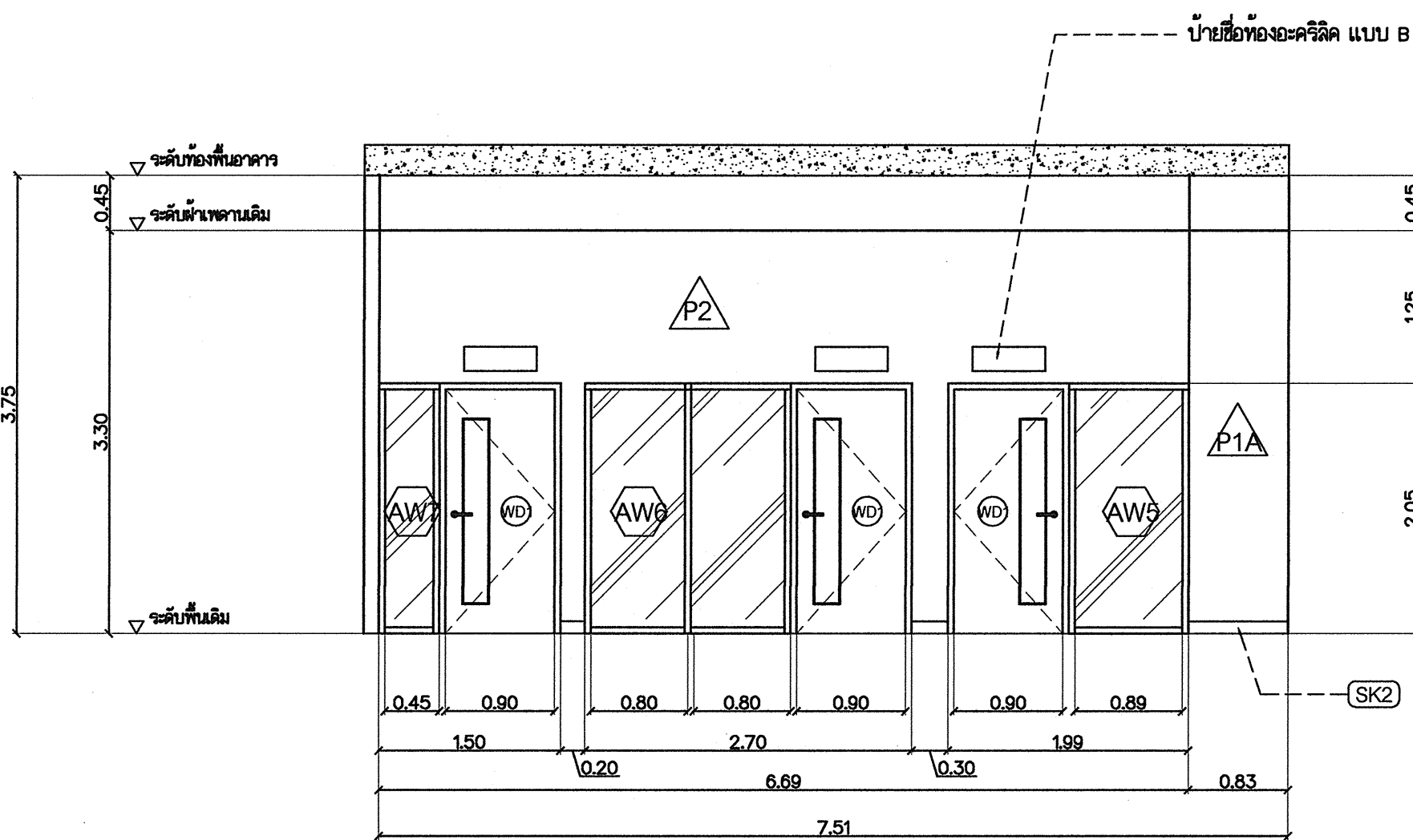
รูปด้าน D SCALE : 1:50
